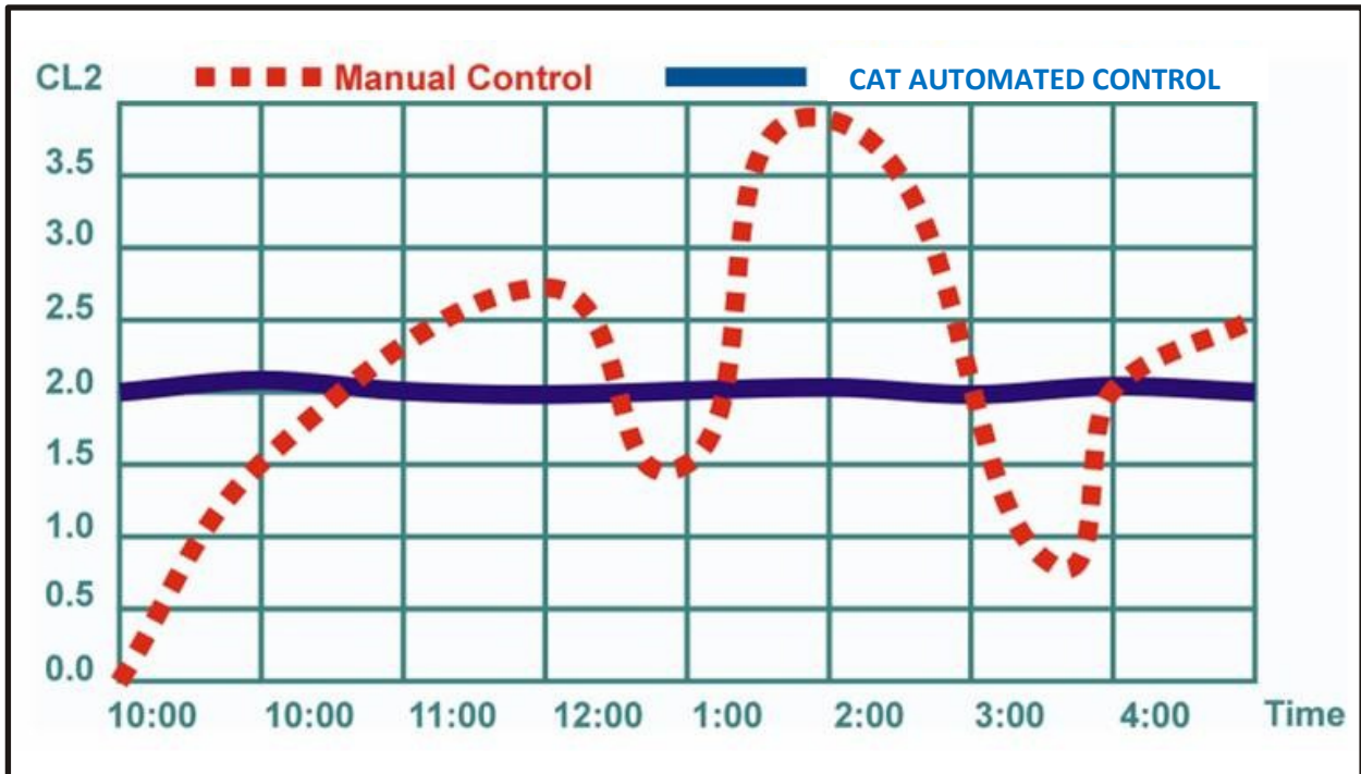
Illustration 1 CONTRÔLE MANUEL COMPARÉ AU CONTRÔLE AUTOMATIQUE
